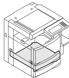
44. DRAWER-ASM
