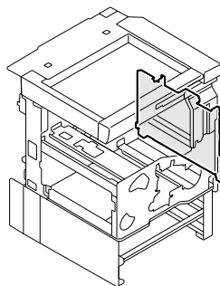
43. ADU-ASM
