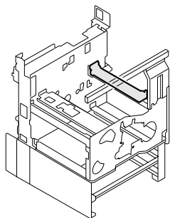
41. FUSER-3-ASM
