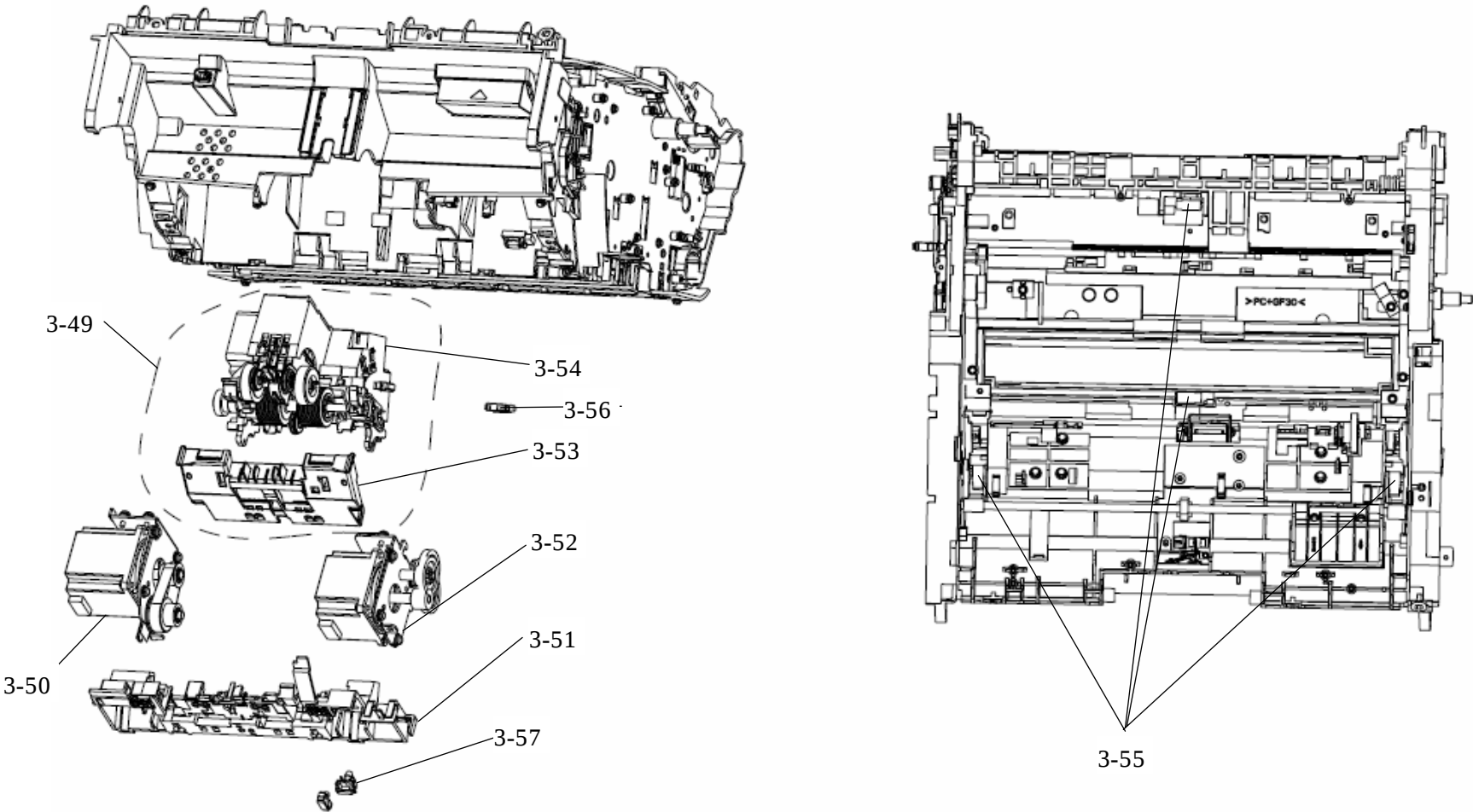
FIGURE3. RV-UNIT 5/5 (-D10 x)
