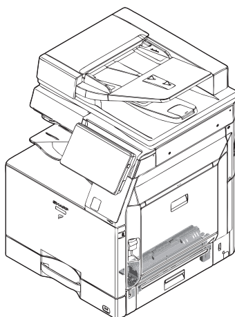
F30-F31 1CS 給紙ユニット (1st Cassette Paper feed unit)
