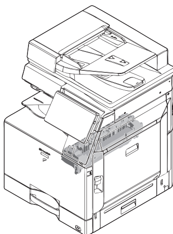
N10 - N12 定着ユニット (Fusing unit)
