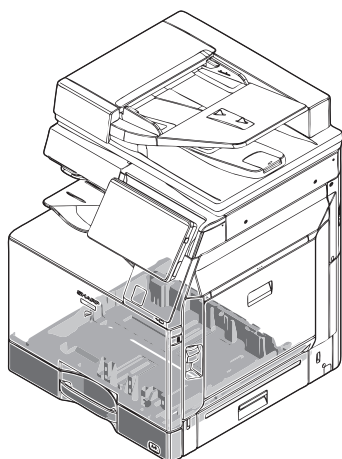
F20 カセットユニット (Cassette unit)
