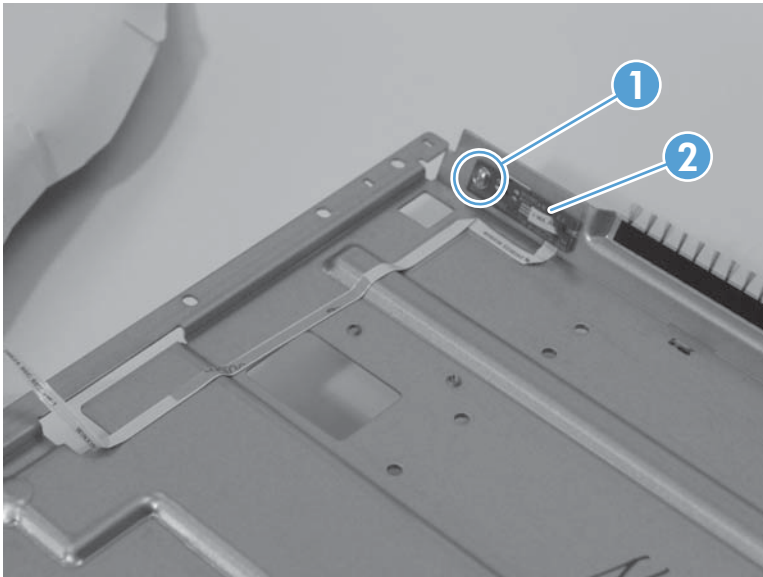
Figure 1-195 Remove the eject flap opto PCA
