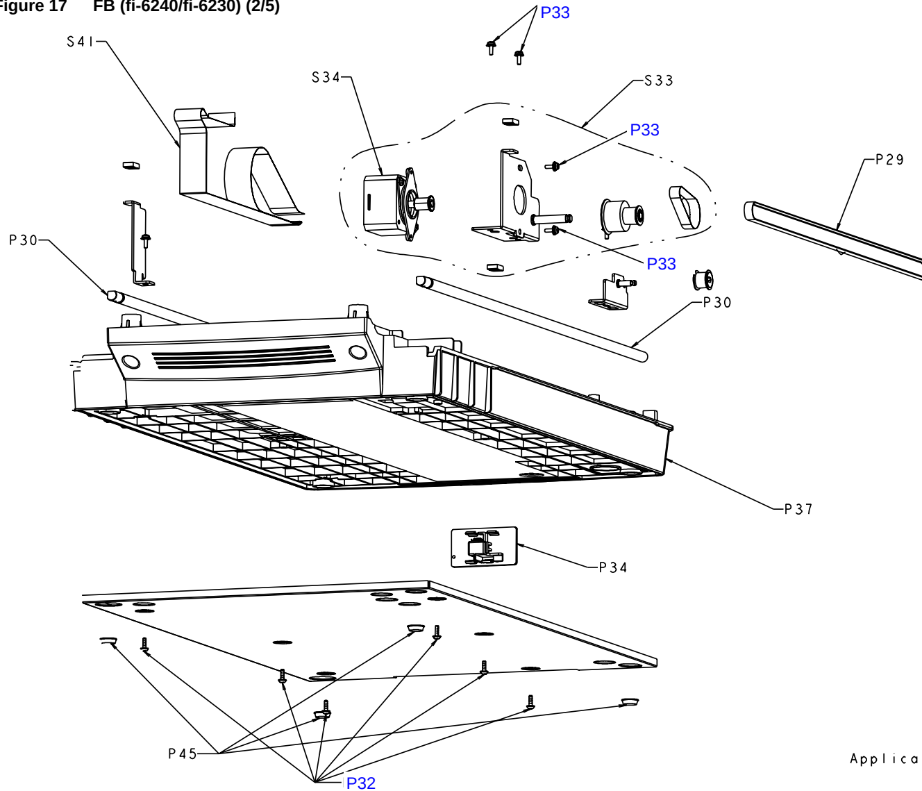
Figure 17 FB (fi-6240/fi-6230) (2/5)
